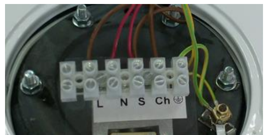
Рис. 3 Фото. Колодка подключения встроенного термостата бойлера STOUT.
